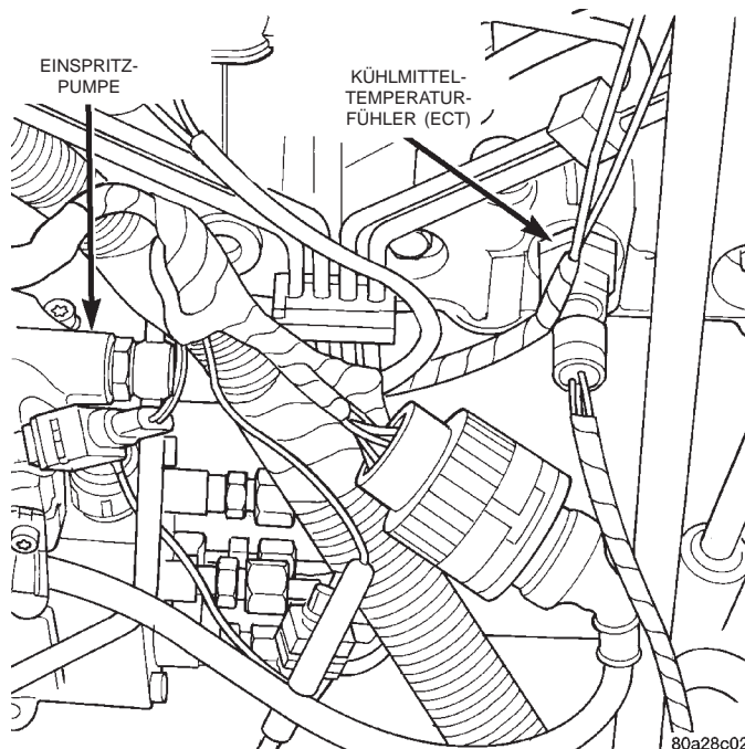
Abb. 14 Lage des Kühlmittel-Temperaturfühlers (ECT)
