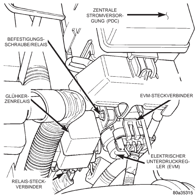
Abb. 11 Lage des Relais
