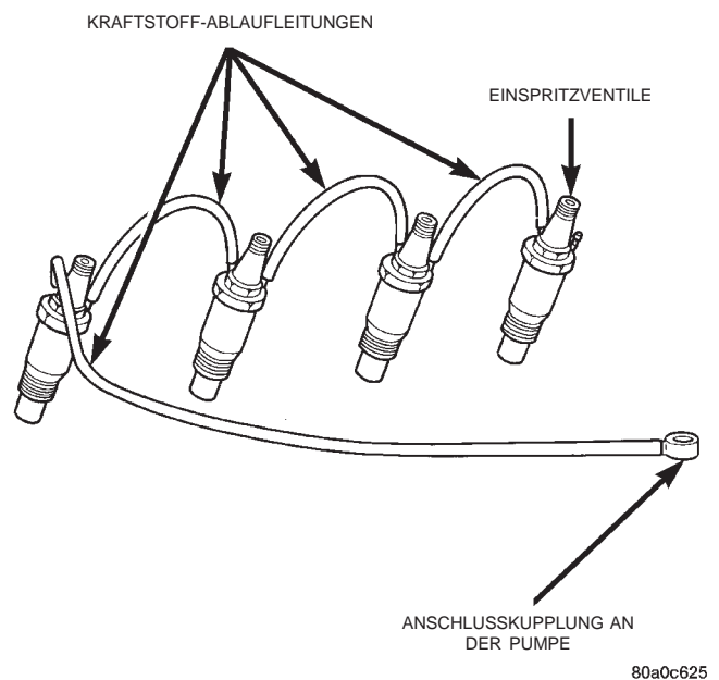
Abb. 6 Einspritzventile und Ablaufleitungen
