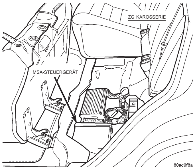
Abb. 2 Lage des MSA-Steuergerätes
