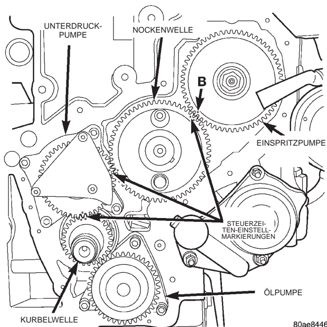
Abb. 21 Unterdruckpumpe an der Motorvorderseite
