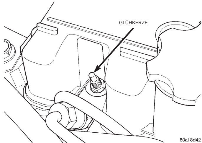
Abb. 13 Glühkerze
