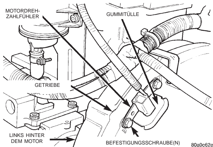
Abb. 19 Motordrehzahlfühler
