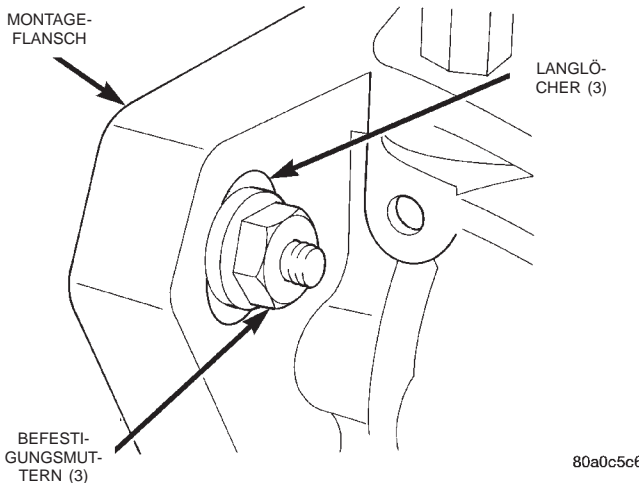
Abb. 38 Befestigungsmuttern der Einspritzpumpe
