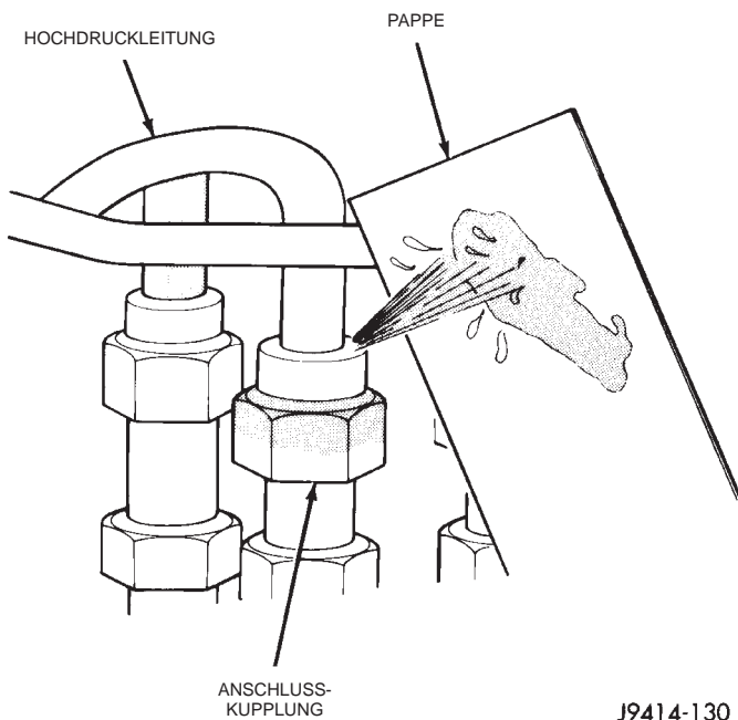
Abb. 24 Beispiel für Leckprüfung mit Pappe
