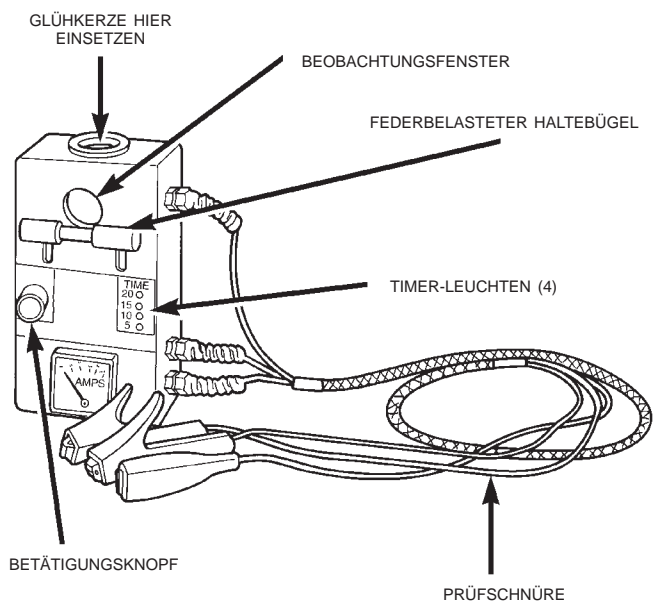
Abb. 15 Beispiel für ein Glühkerzen-Testgerät
