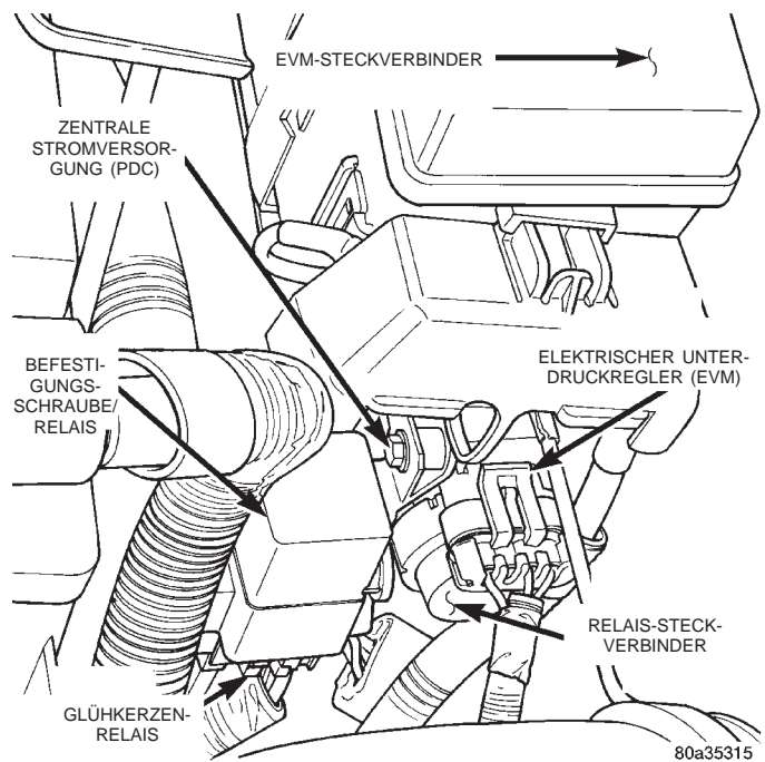
Abb. 23 Lage des Glühkerzenrelais
