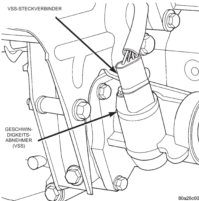
Abb. 8 Geschwindigkeitsabnehmer (VSS)—Beispiel
