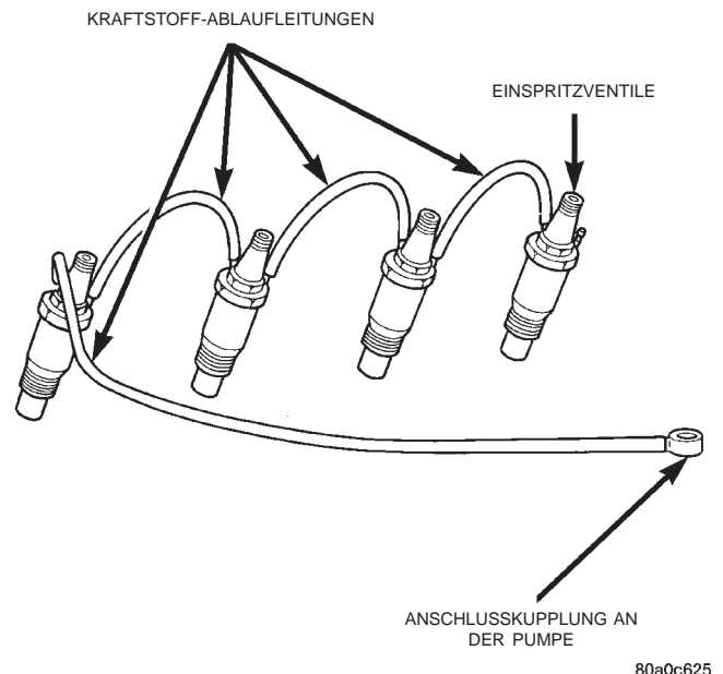
Abb. 9 Kraftstoff-Ablaufleitungen
