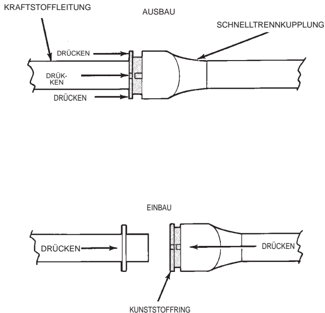
Abb. 8 Kupplung mit Kunststoffhalterung
