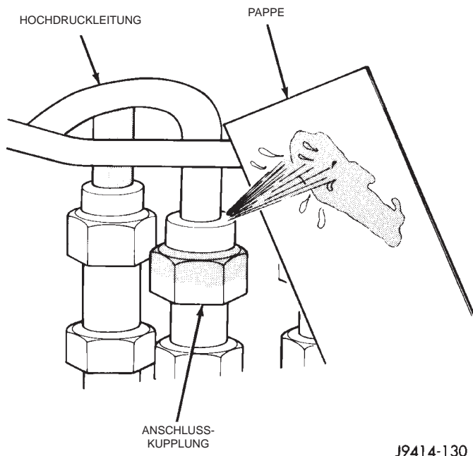
Abb. 1 Beispiel für Kraftstoff-Drucktest am Einspritzventil
