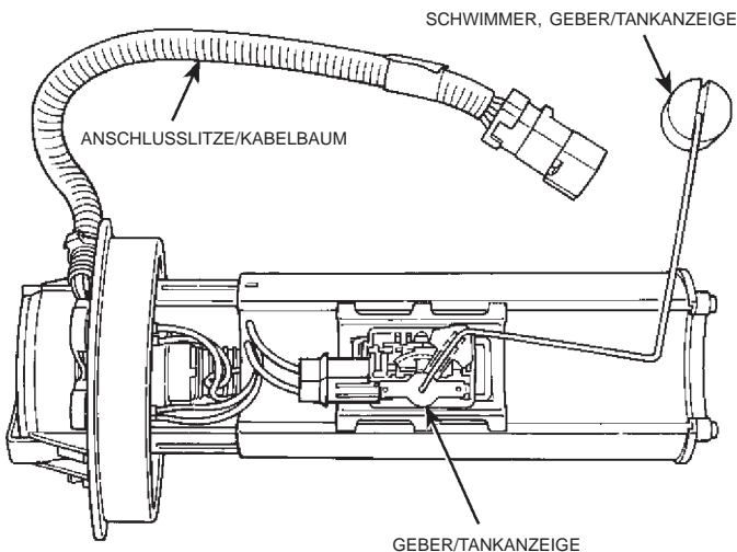
Abb. 31 Geber/Tankanzeige
