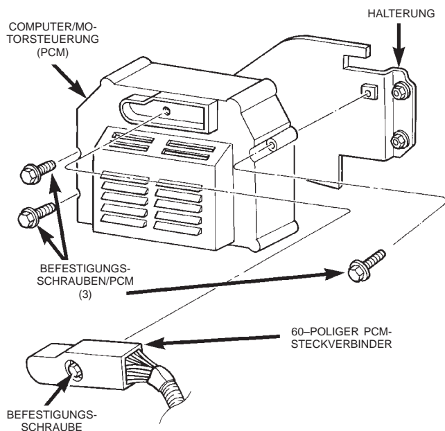
Abb. 1 Lage des PCM
