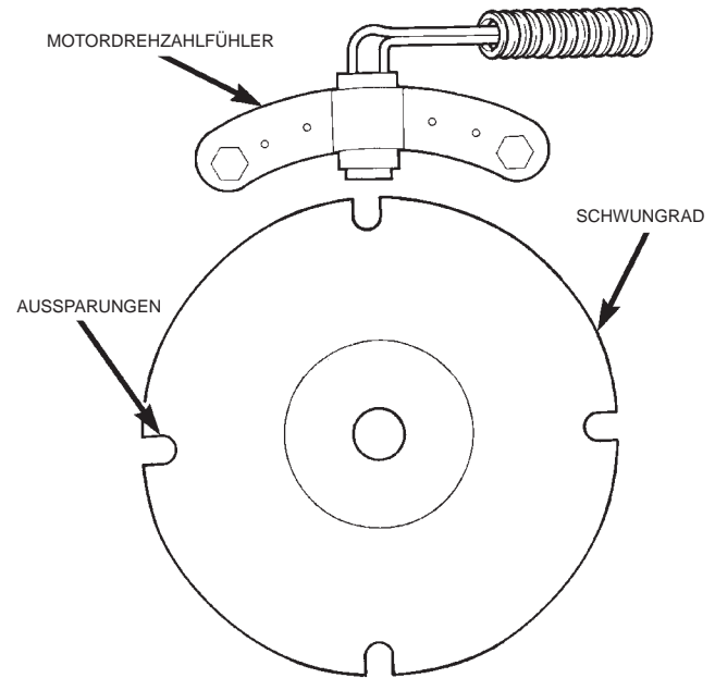
Abb. 6 Funktionsweise des Drehzahlfühlers
