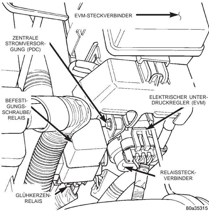
Abb. 30 Lage der zentralen Stromversorgung (PDC)
