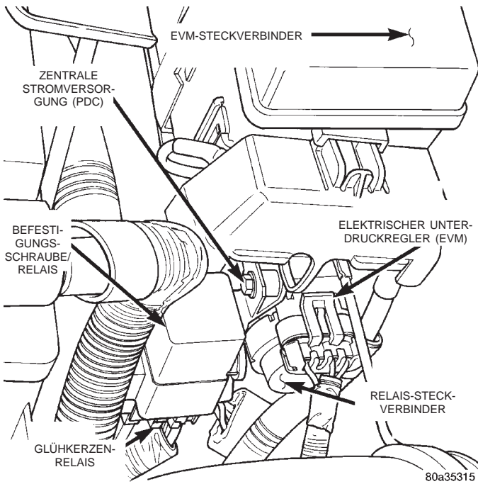
Abb. 12 Lage des Glühkerzenrelais
