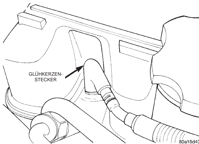
Abb. 17 Leitungsanschluß an der Glühkerze
