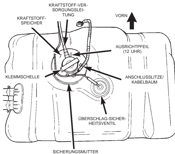
Abb. 2 Kraftstoffbehälter
