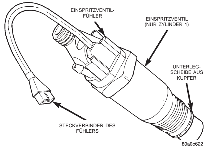
Abb. 3 Einspritzventilfühler
