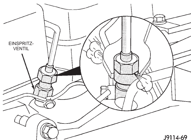
Abb. 26 Hochdruck-Kraftstoffleitung entlüften— Beispiel
