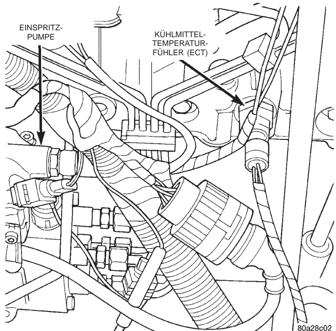
Abb. 4 Lage des Kühlmittel-Temperaturfühlers (ECT)
