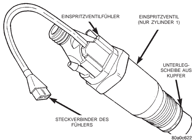
Abb. 23 Lage des Einspritzventilfühlers
