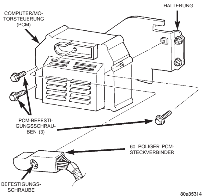
Abb. 12 Lage des PCM — Beispiel
