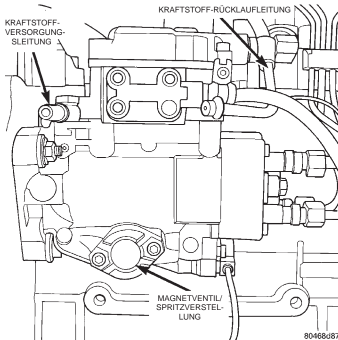
Abb. 11 Magnetventil/Spritzverstellung
