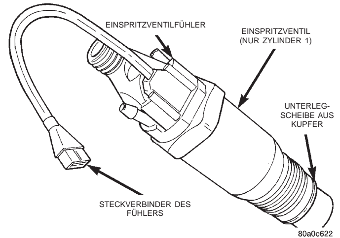
Abb. 17 Einspritzventilfühler
