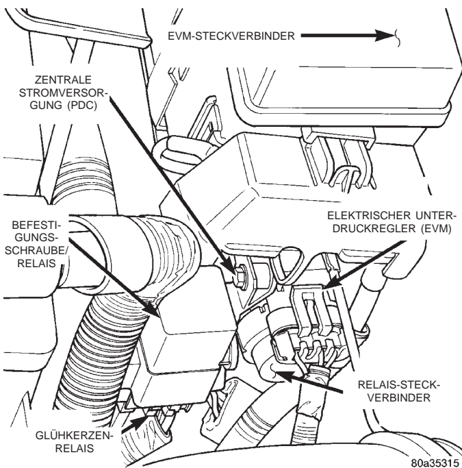
Abb. 18 ASD-Relais und andere Relaissteckplätze
