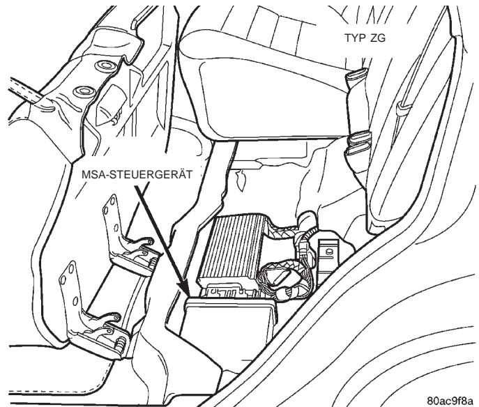
Abb. 13 Lage des MSA-Steuergeräts — Beispiel
