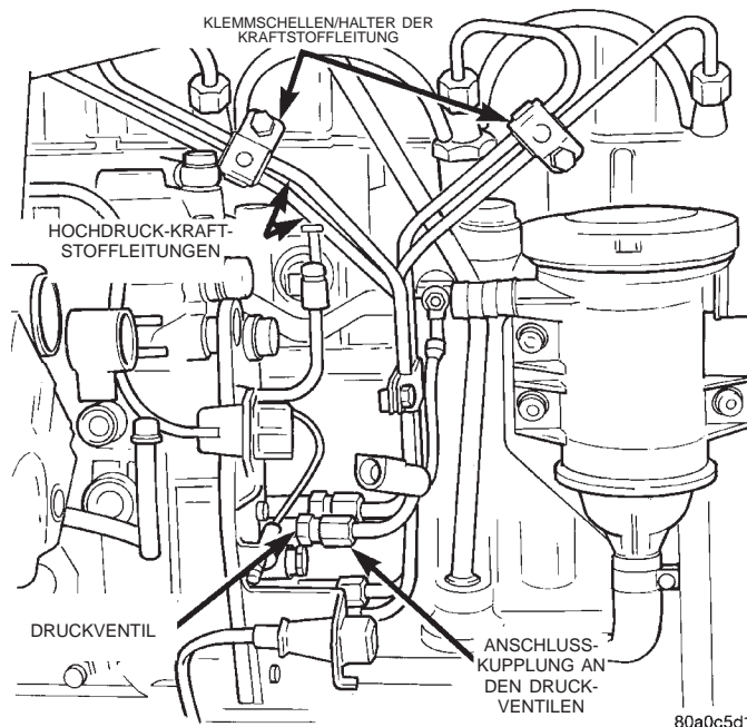
Abb. 48 Kraftstoffleitungen und Klemmschellen/Halter
