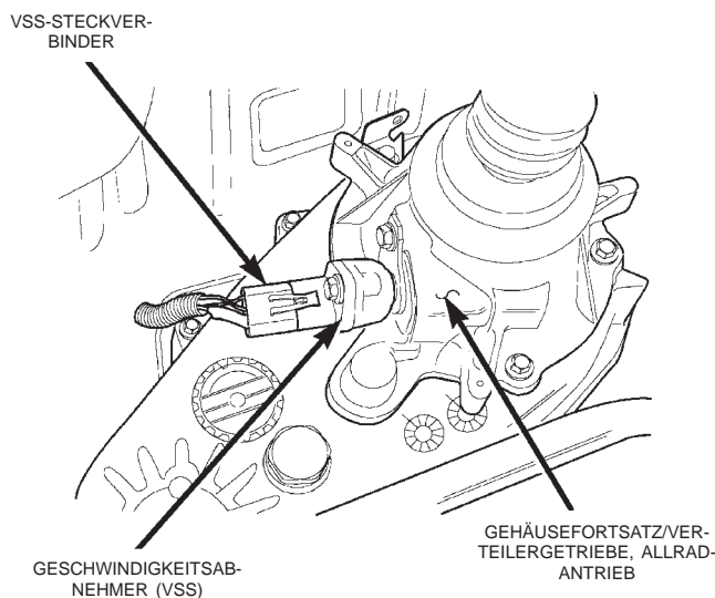
Abb. 25 Lage des Geschwindigkeitsabnehmers (VSS) — Fahrzeuge mit Hinterradantrieb
