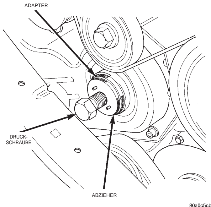
Abb. 37 Montage der Ausbauwerkzeuge für das Antriebsrad
