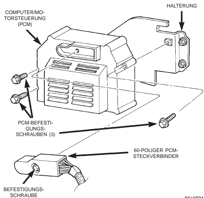
Abb. 2 Lage des Computers/Motorsteuerung (PCM)
