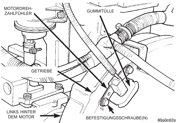
Abb. 5 Lage des Motordrehzahlfühlers
