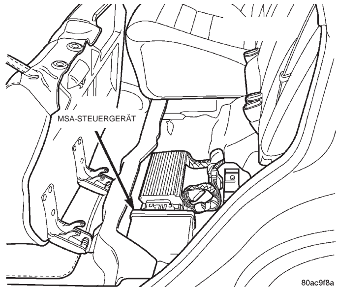
Abb. 1 Lage des MSA-Steuergeräts
