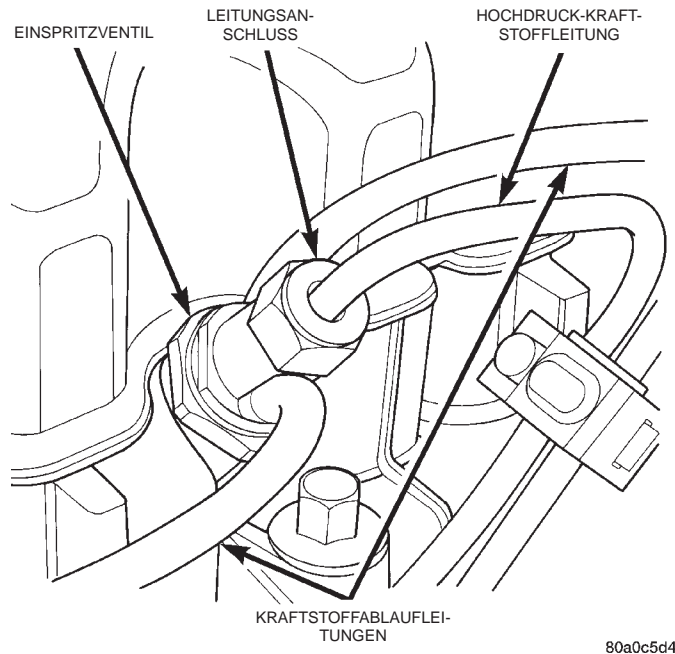
Abb. 42 Einspritzventil—Beispiel
