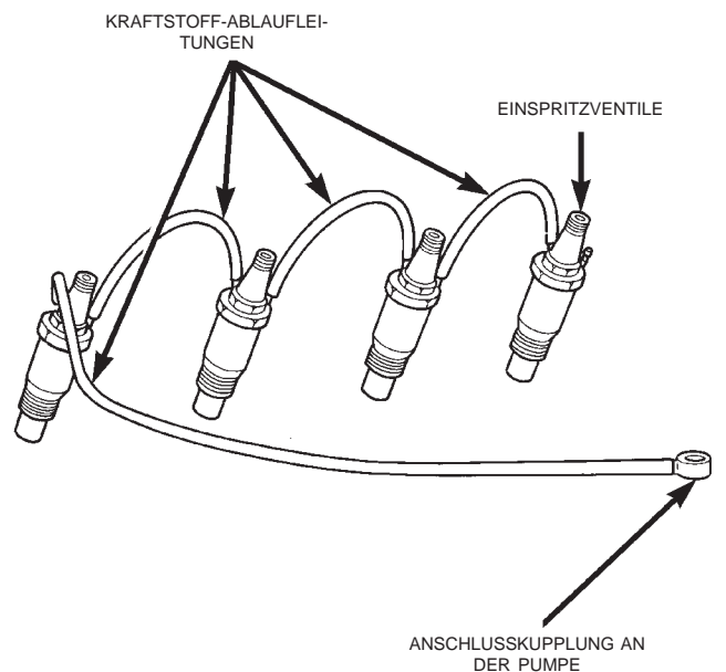
Abb. 28 Kraftstoff-Ablaufleitungen
