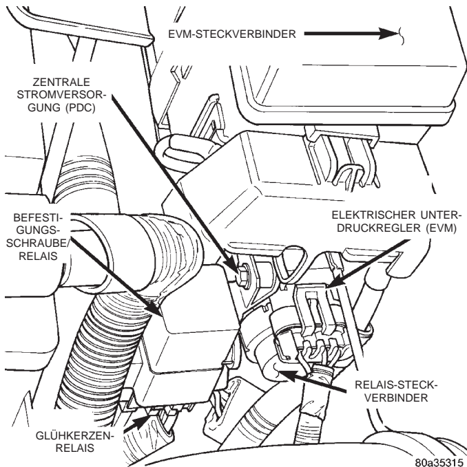
Abb. 16 Lage des Glühkerzenrelais
