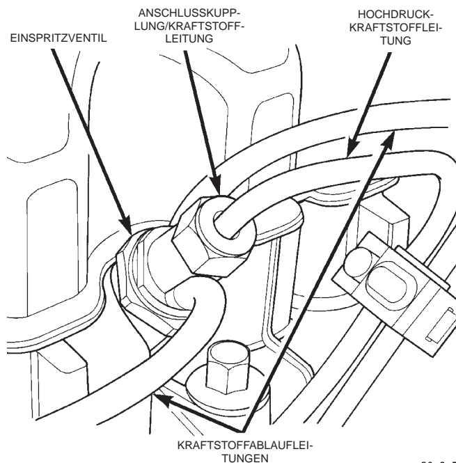
Abb. 49 Kraftstoffleitungen an den Einspritzventilen eingebaut werden, in der sie ausgebaut wurden! Die Halter der Druckventile der Einspritzpumpe (Abb. 48) dürfen sich beim Aus- oder Einbau der Hochdruckleitungen von der Einspritzpumpe nicht drehen.
