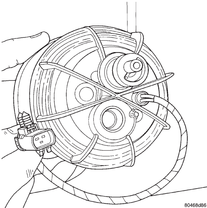
Abb. 10 Lage des Temperaturfühlers/ Kraftstoffvorwärmung und des Kraftstoff- Heizelementes
