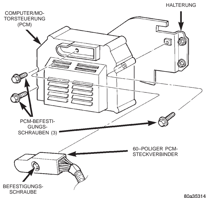
Abb. 24 Lage des PCM
