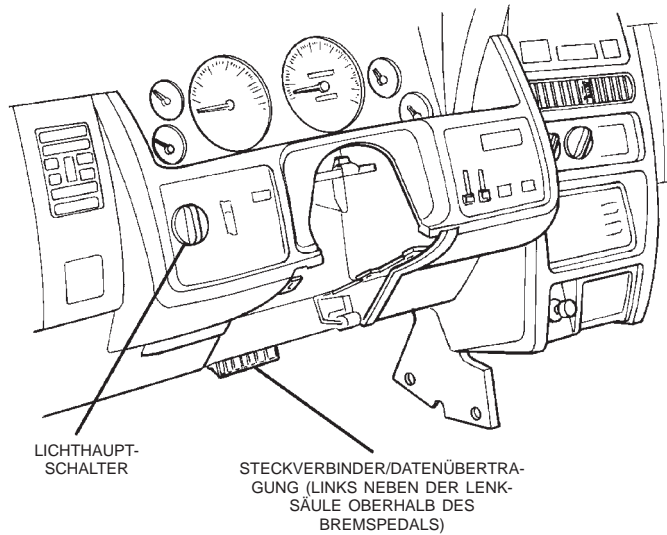
Abb. 7 Lage des Steckverbinders/Datenübertragung GESCHWINDIGKEITSABNEHMER (VSS) — EINGANGSSIGNAL/MSA
