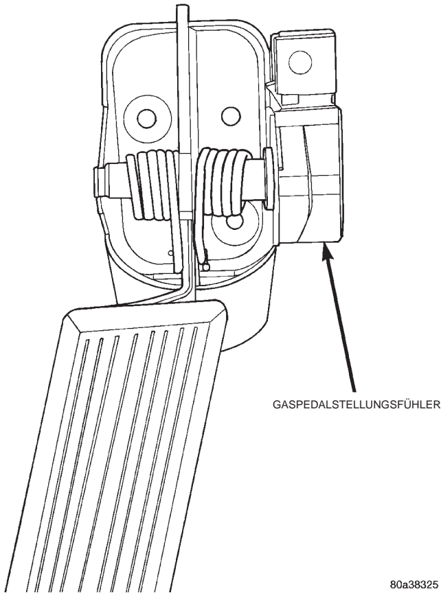
Abb. 27 Gaspedalbefestigung - Beispiel
