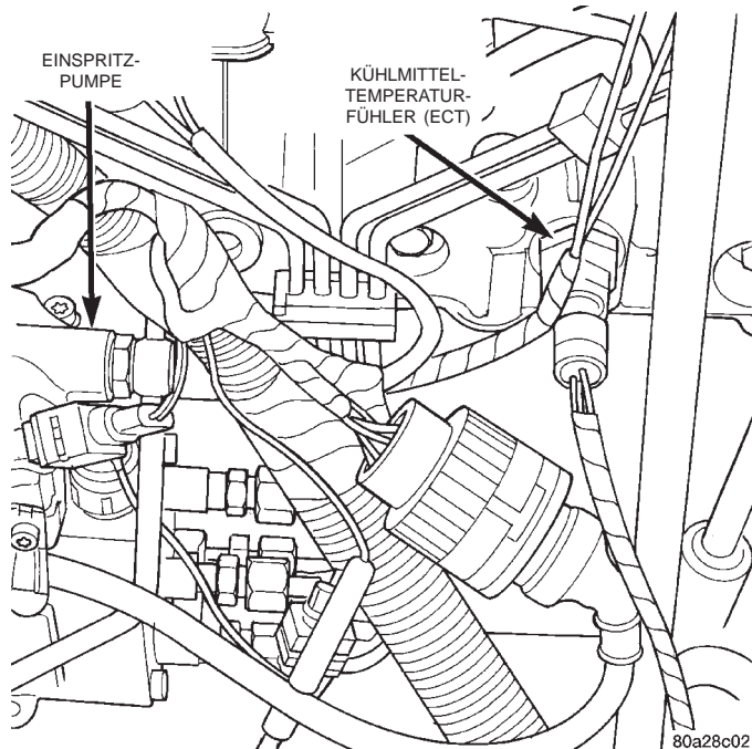
Abb. 20 Lage des Kühlmittel-Temperaturfühlers (ECT)
