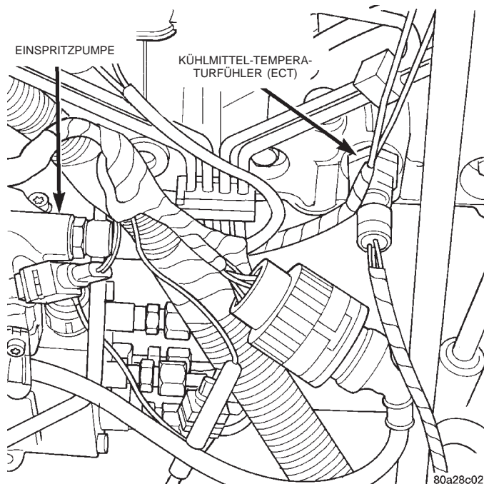
Abb. 20 Lage des Kühlmittel-Temperaturfühlers (ECT)
