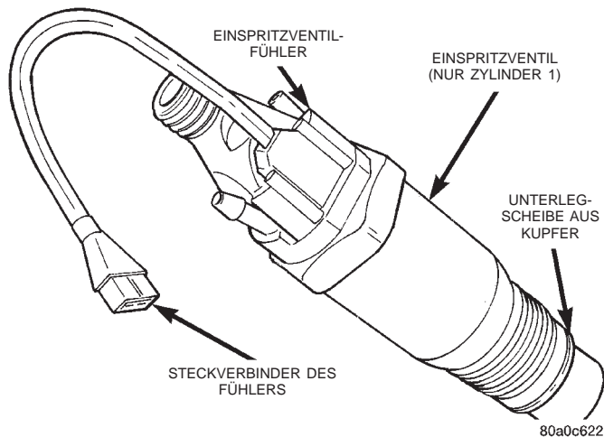
Abb. 7 Einspritzventilfühler
