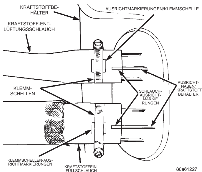
Abb. 45 Ausrichtmarkierungen, Kraftstoffeinfüllschlauch/Entlüftungsschlauch
