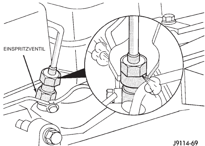
Abb. 22 Beispiel für Prüfung eines Einspritzventils
