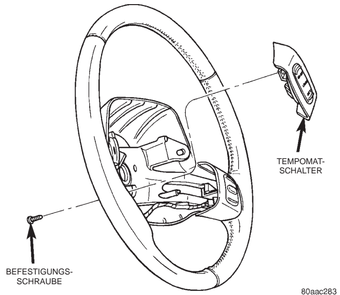
Abb. 4 Tempomat-Schalter aus- und einbauen
