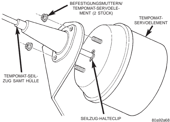
Abb. 3 Clip des Tempomat-Servolements aus- und einbauen—Typisch
