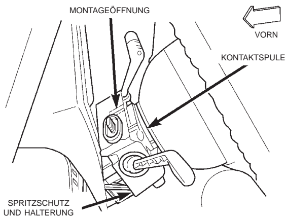
Abb. 22 Montageöffnung im Spritzschutz des Kombischalters
